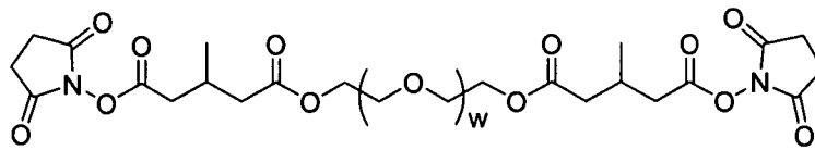
PEG 3350 -S3MG
