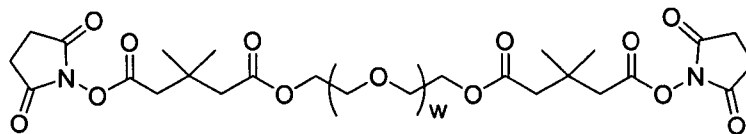
PEG 3350 -S3,3DMG
